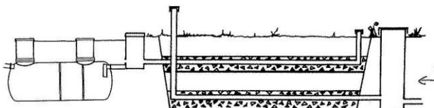
Renat avloppsvatten leds ut till dike
