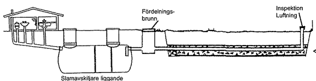
Renat avloppsvatten sugs upp i mark
